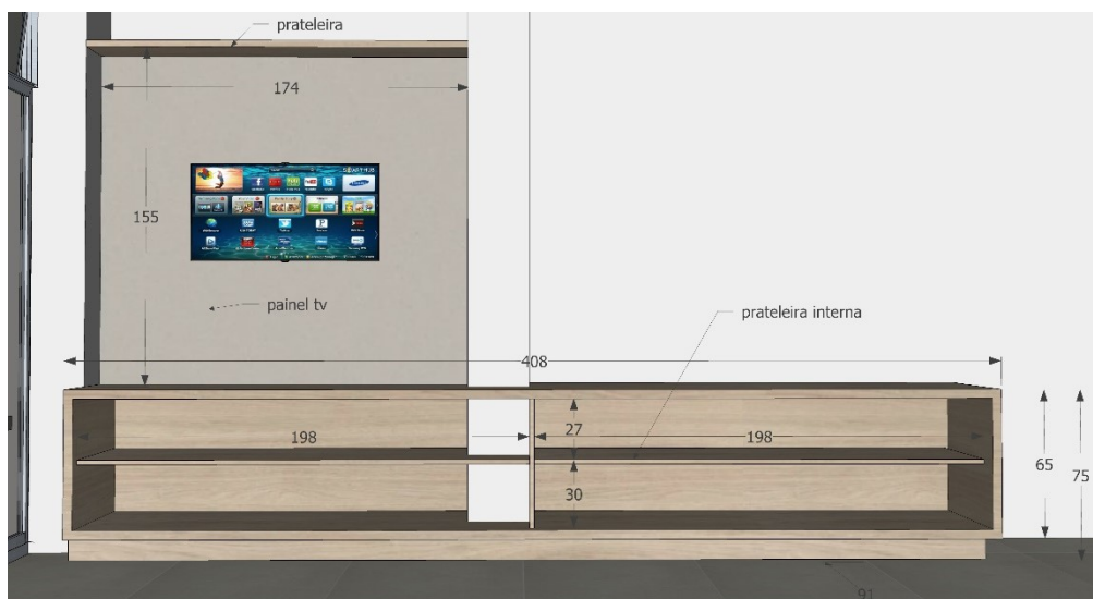
Imagem 08 – Layout Mobiliário Sala Secretária
