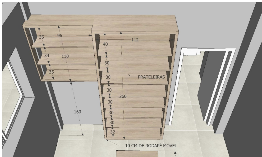
Imagem 14 – Detalhamento Móvel – Sala Administrativa 01
