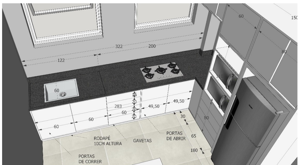
Imagem 32 – Detalhamento Mobiliário – Cozinha
