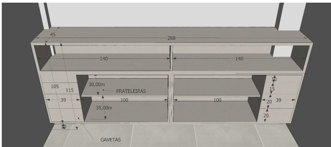
Imagem 21 – Detalhamento Mesas – Sala Administrativa 02
