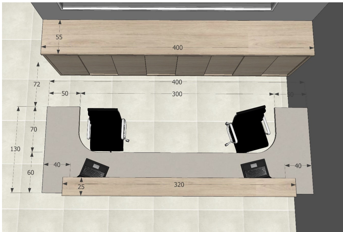
Imagem 01 – Layout Mobiliário Recepção
