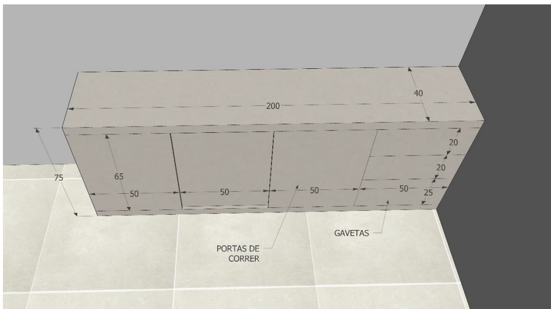
Imagem 15 – Detalhamento Mesa – Sala Administrativa 01
