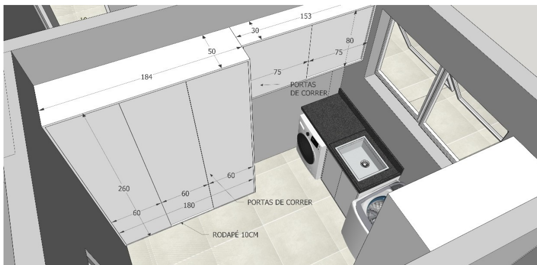
Imagem 25 – Detalhamento Mobiliário – Lavadeira
