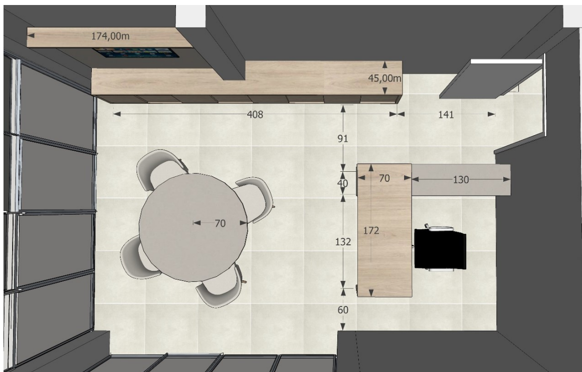
Imagem 06 – Layout Mobiliário Sala Secretária
