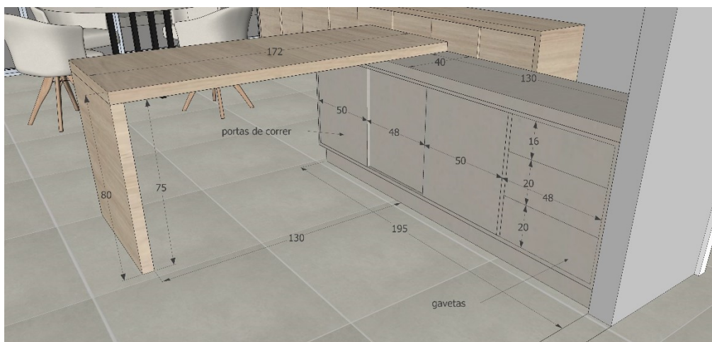
Imagem 09 – Detalhamento mesas secretária
