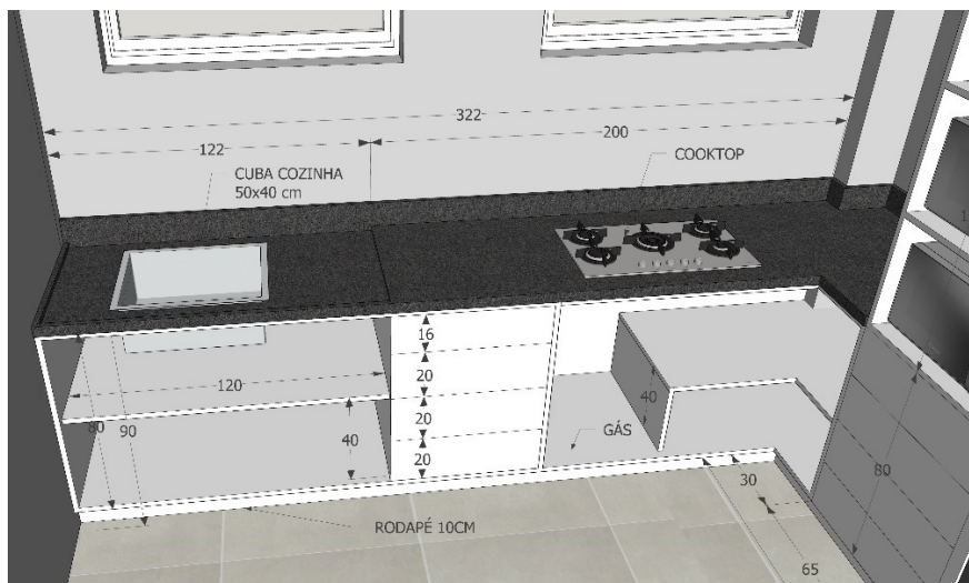
Imagem 33 – Detalhamento Mobiliário – Cozinha
