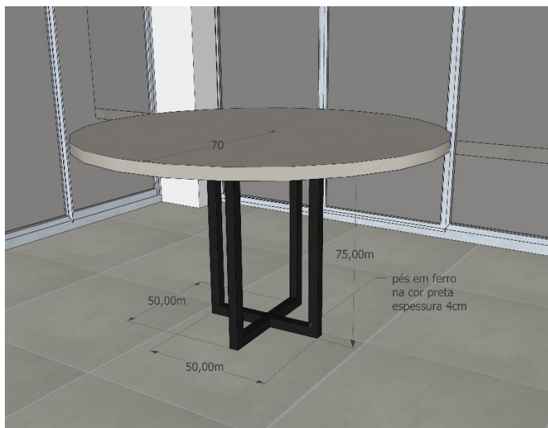
Imagem 11 – Detalhamento mesa de reunião
