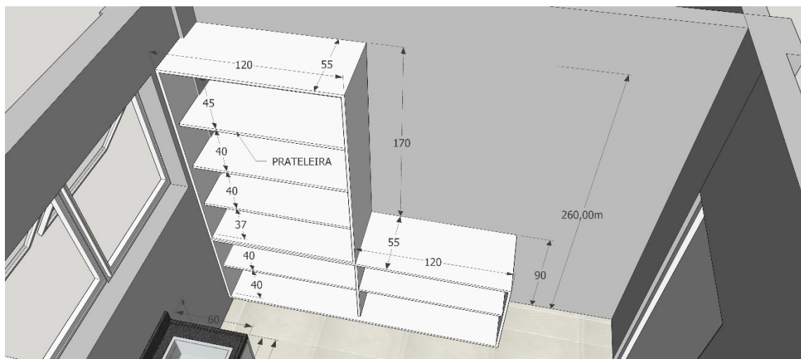
Imagem 29 – Detalhamento Mobiliário – Lavadeira
