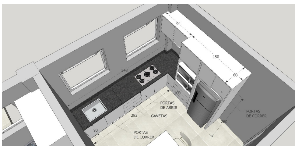
Imagem 31 – Detalhamento Mobiliário – Cozinha
