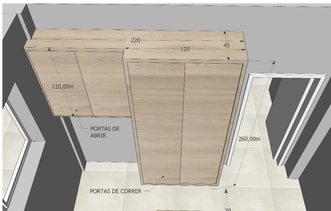
Imagem 13 – Detalhamento Móvel – Sala Administrativa 01
