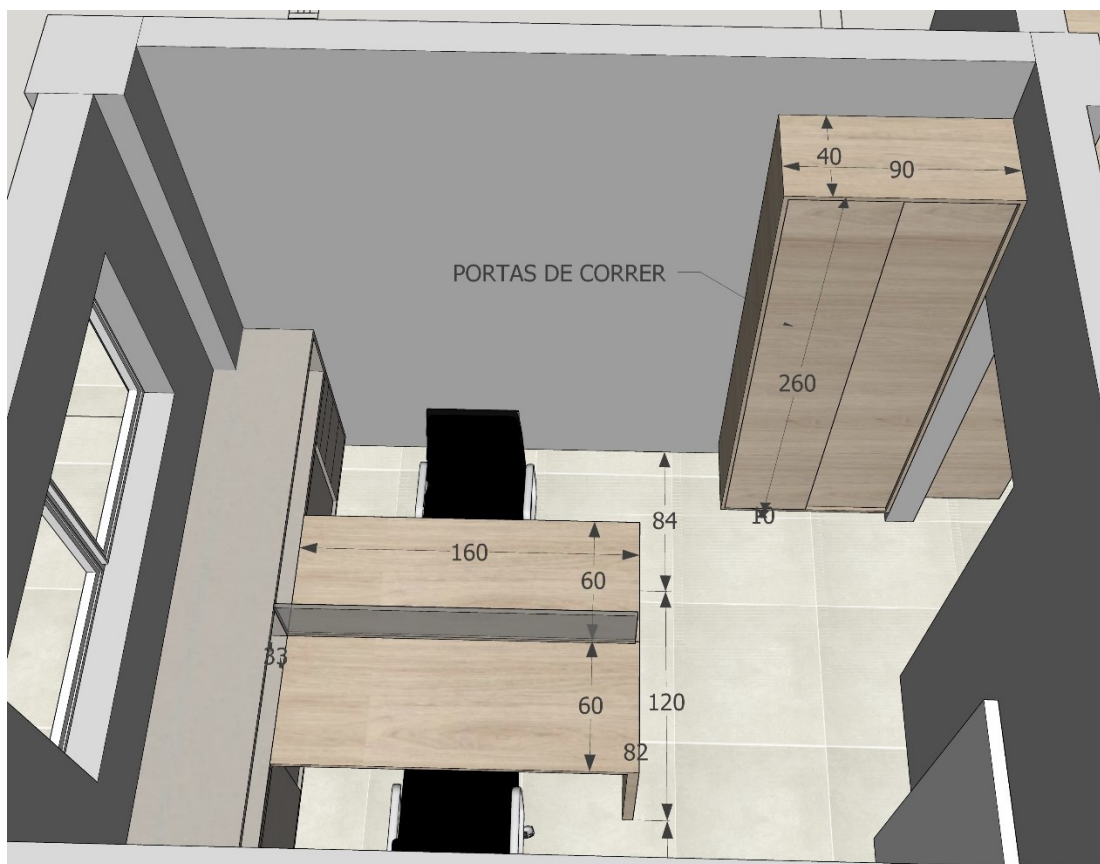
Imagem 16 – Detalhamento – Sala Administrativa 02
