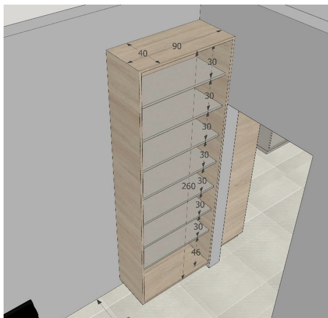
Imagem 17 – Detalhamento Armário – Sala Administrativa 02
