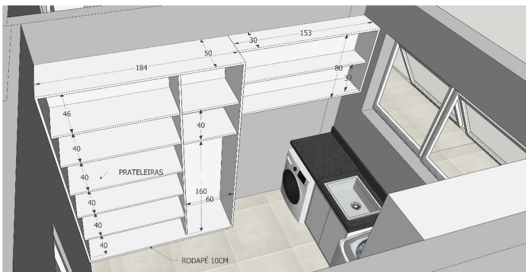
Imagem 26 – Detalhamento Mobiliário – Lavadeira
