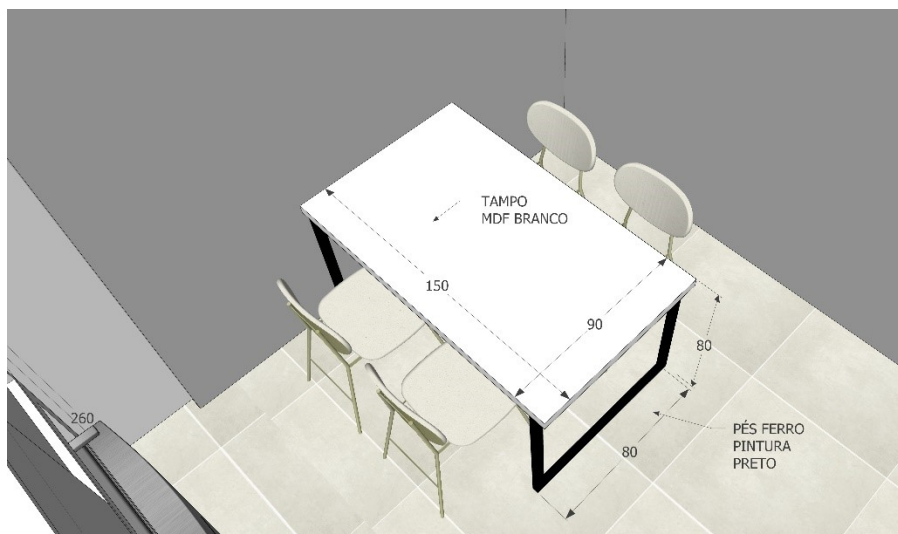
Imagem 35 – Detalhamento Mobiliário – Cozinha
