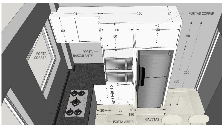
Imagem 34 – Detalhamento Mobiliário – Cozinha
