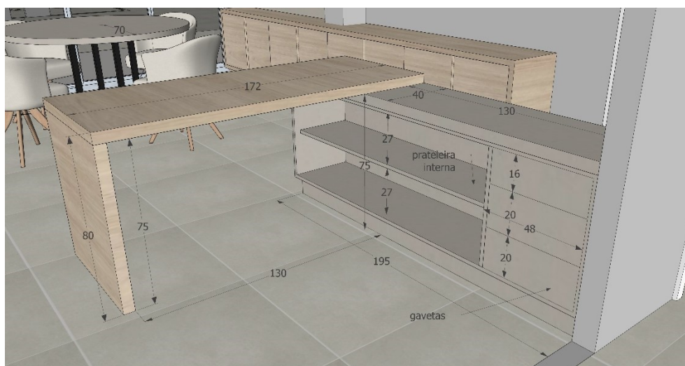
Imagem 10 – Detalhamento mesas secretária
