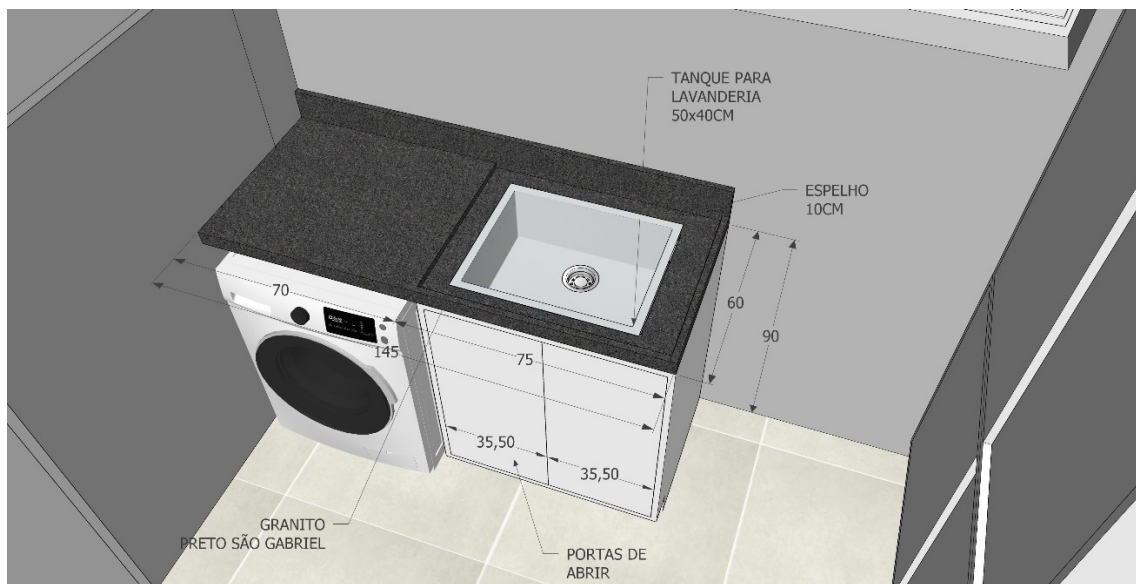
Imagem 27 – Detalhamento Mobiliário – Lavadeira
